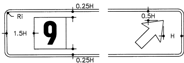
Sinal de pré-aviso simplificado
