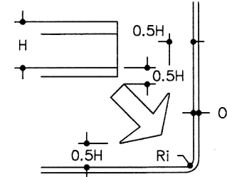
Painéis em pórtico
