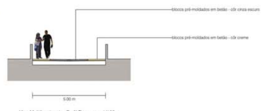
Vias Multifuncionais Perfil Tipo - esc. 1/100
